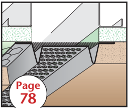
SBS: BugStop® Soffit Vent
